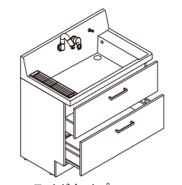
フルスライドタイプ AR3FH-905SY
